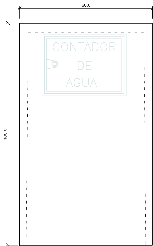
ALZADO
